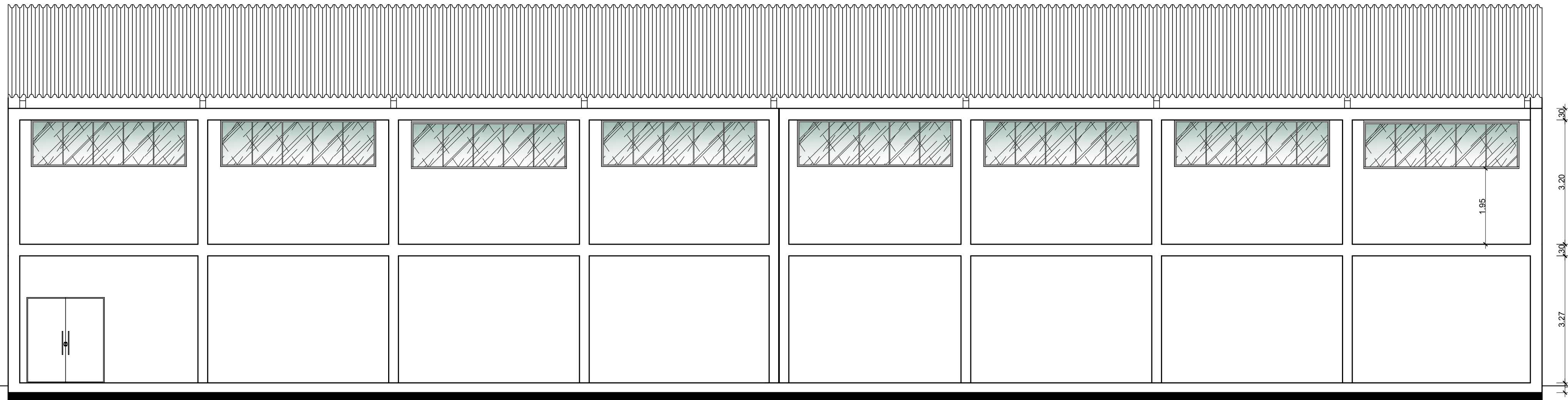
02 FACHADA FUNDOS ESCALA 1/75
