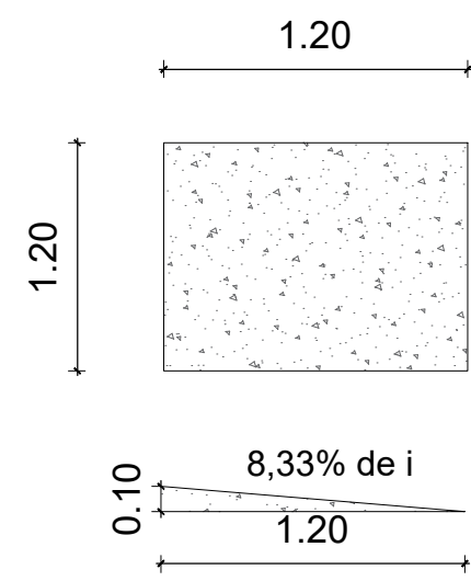
Detalhamento rampa
