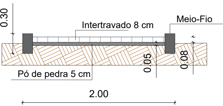
Detalhamento pavimentação
