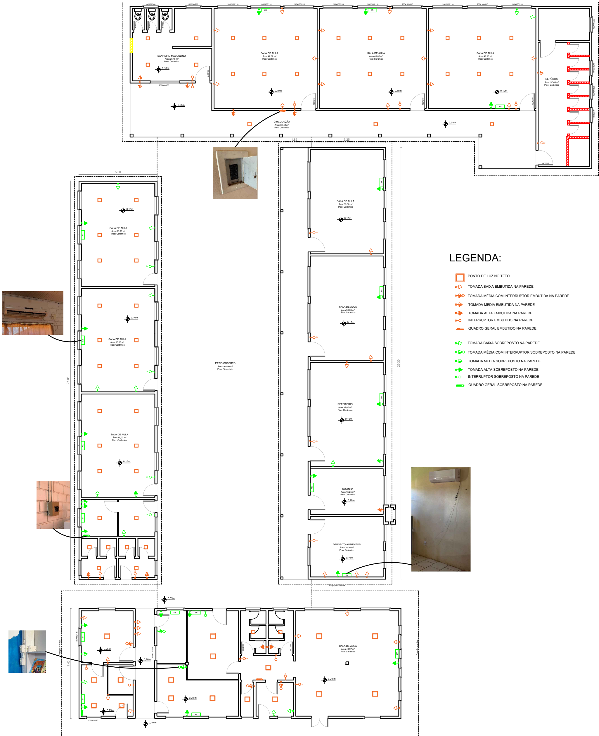
PLANTA BAIXA TÉCNICA - SITUAÇÃO ATUAL - ELÉTRICO A = m² / Escala = 1 : 150
